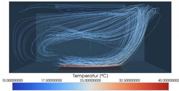
Abbildung 7: Stromlinien Open-FOAM-Berechnung
